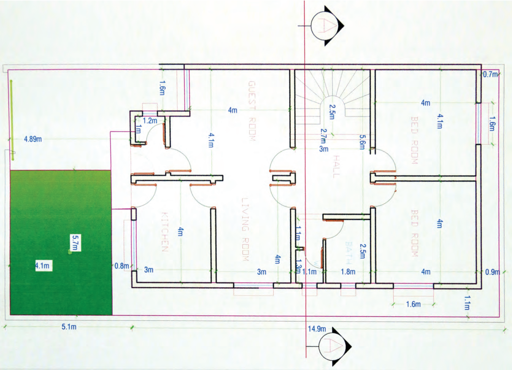
خريطة الوحدة السكنية
